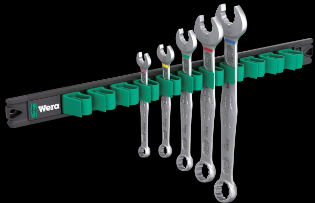
环形扳手组套, 公制尺寸, 扳手开口的回转角为 7.5° 5 件组套 在接线盒上
